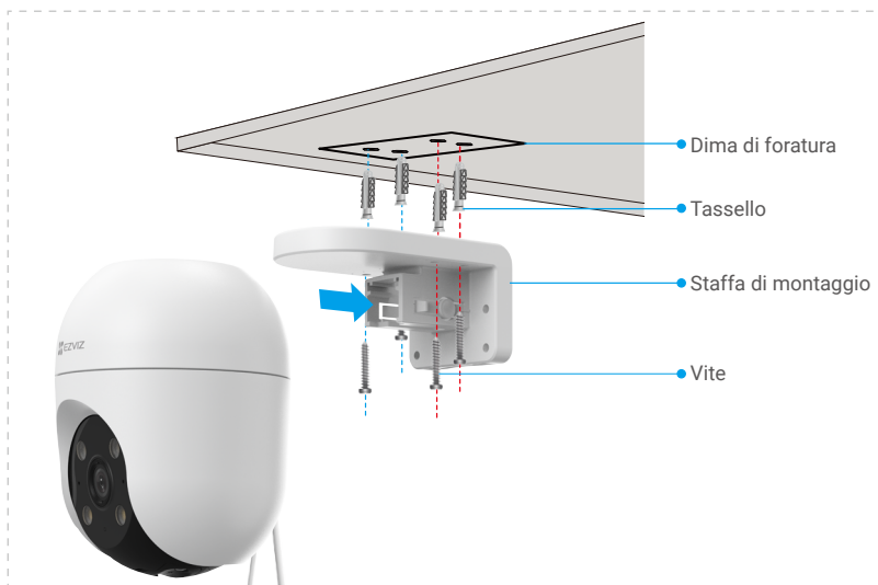
Fig. 1 Montaggio a soffitto
