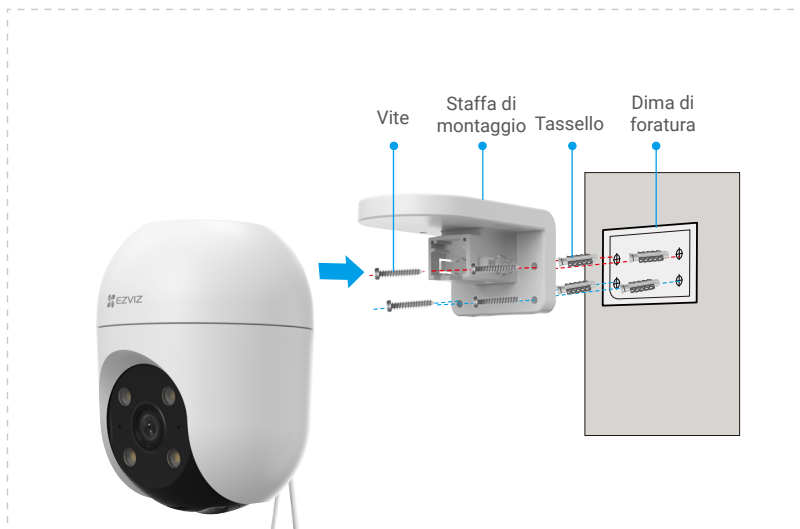
Fig. 2 Montaggio a parete
